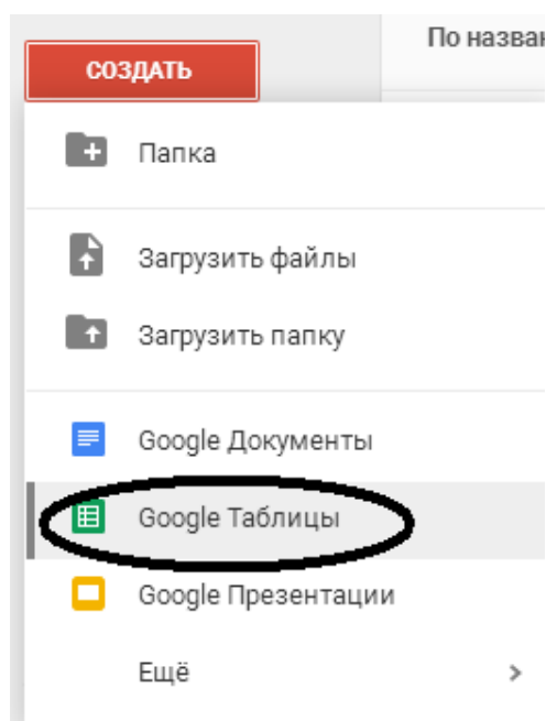
Рисунок 3. Меню Создать.
