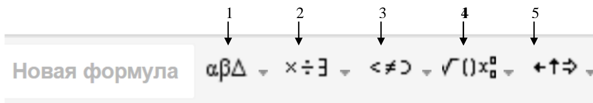
Рисунок 12. Панель формул.
